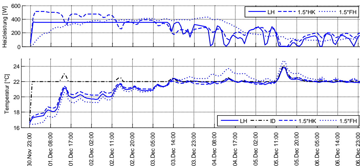
Abbildung 31: Aufheizverhalten des Wohnzimmers nach „Erstbezug“ im Dezember für Referenzfall aber mit 1,5-facher Heizleistungs-Auslegung (480 W statt 300 W) für Heizkörper und Fußbodenheizung. Dies soll die in der Realität oft umgesetzte „Überdimensionierung“ der Heizflächen abbilden.
