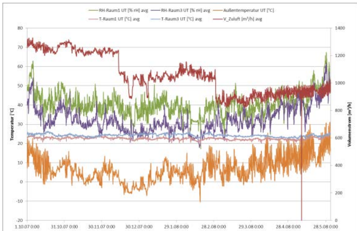
Abbildung 78: Analyse der Raumlufftfeuchte in Raum1 und Raum3
