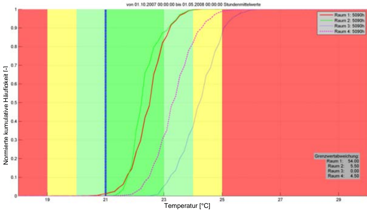
Abbildung 75: Utendorfsgasse, Heizperiode (1. Oktober – 30. April), Werte rechts oben stellen die Gesamtstundenzahl der gemessenen Werte für jeden Raum dar, Zielwertabweichung stellt die gewichtete Stundenzahl unter 21°C dar
