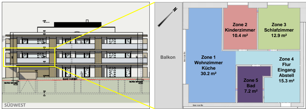
Abbildung 4: Außenansicht und Grundriss der gewählten Referenzwohnung. Für die dynamische Gebäudesimulation wurde die Wohnung in fünf Temperaturzonen unterteilt.
