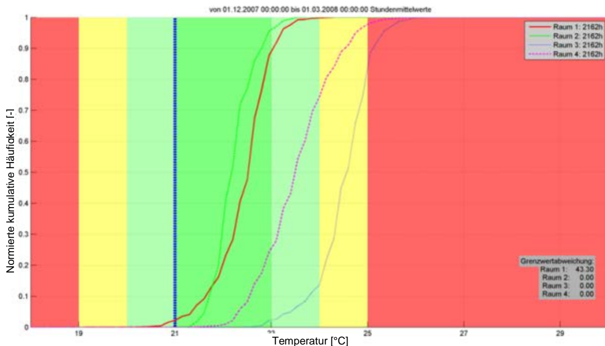
Abbildung 74: Utendorfasse, Kernwinter (1. Dezember – 28. Februar), Werte rechts oben stellen die Gesamtstundenzahl der gemessenen Werte für jeden Raum dar, die Zielwertabweichung stellt die gewichtete Stundenzahl unter 21°C dar
