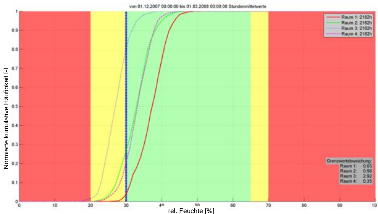
Abbildung 76: Utendorfsgasse, Kernwinter (1. Dezember – 28. Februar), Werte rechts oben stellen die Gesamtstundenzahl der gemessenen Werte für jeden Raum dar, Zielwertabweichung stellt die Summe der Unterschreitung der Grenze von 30 %-rF dar
