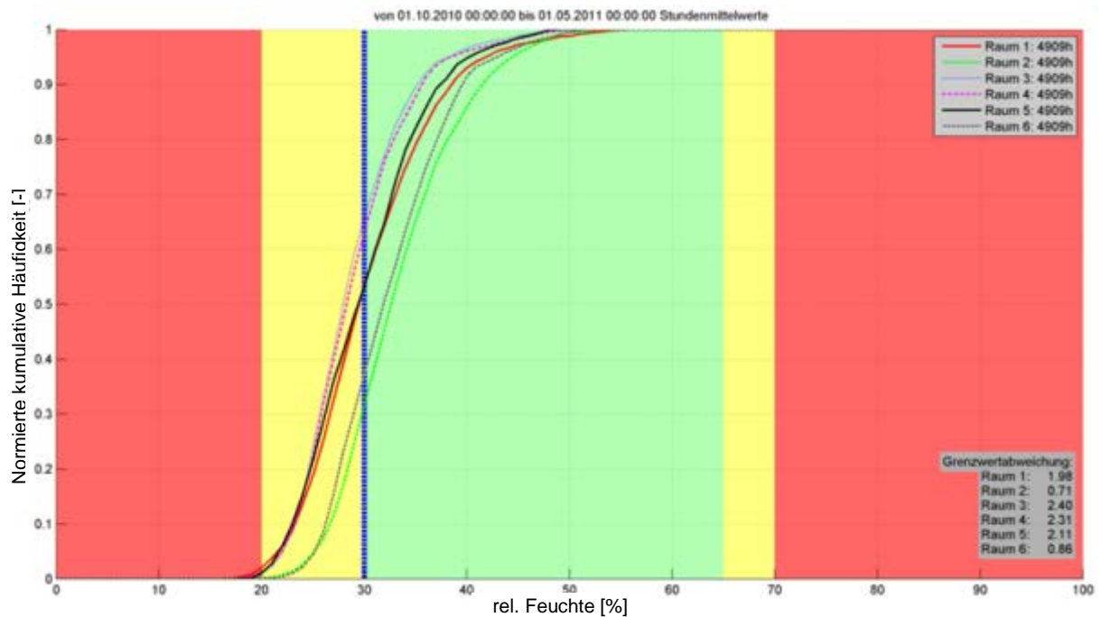
Abbildung 111: Lodenareal, Heizperiode (1. Oktober – 30. April) W7-12, Werte rechts oben stellen die Gesamtstundenzahl der gemessenen Werte für jeden Raum dar, Zielwertabweichung stellt die Summe der Unterschreitung der Grenze von 30 %-rF dar
