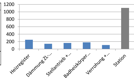
Abbildung 64: Kostenzusammenstellung für eine Luftheizung für die Referenzwohnung.
