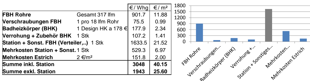
Abbildung 63: Kostenzusammenstellung für eine Fußbodenheizung für die Referenzwohnung.
