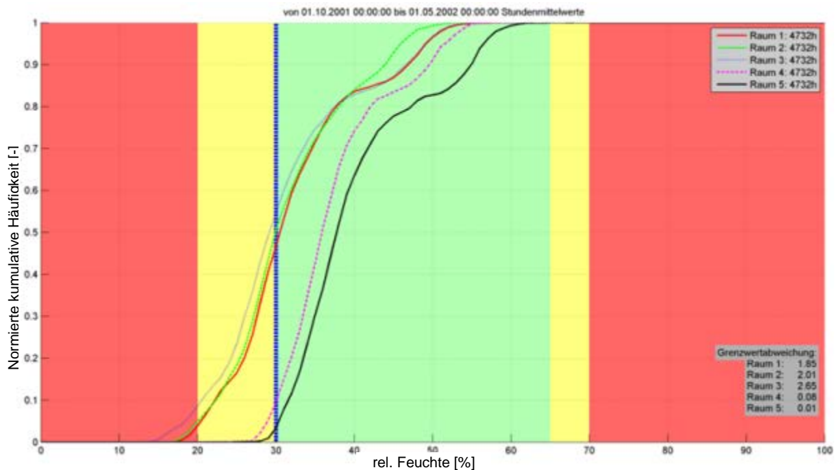
Abbildung 89: Wolfurt, Heizperiode (1. Oktober – 30. April), Werte rechts oben stellen die Gesamtstundenzahl der gemessenen Werte für jeden Raum dar, Zielwertabweichung stellt die Summe der Unterschreitung der Grenze von 30 % rF dar.
