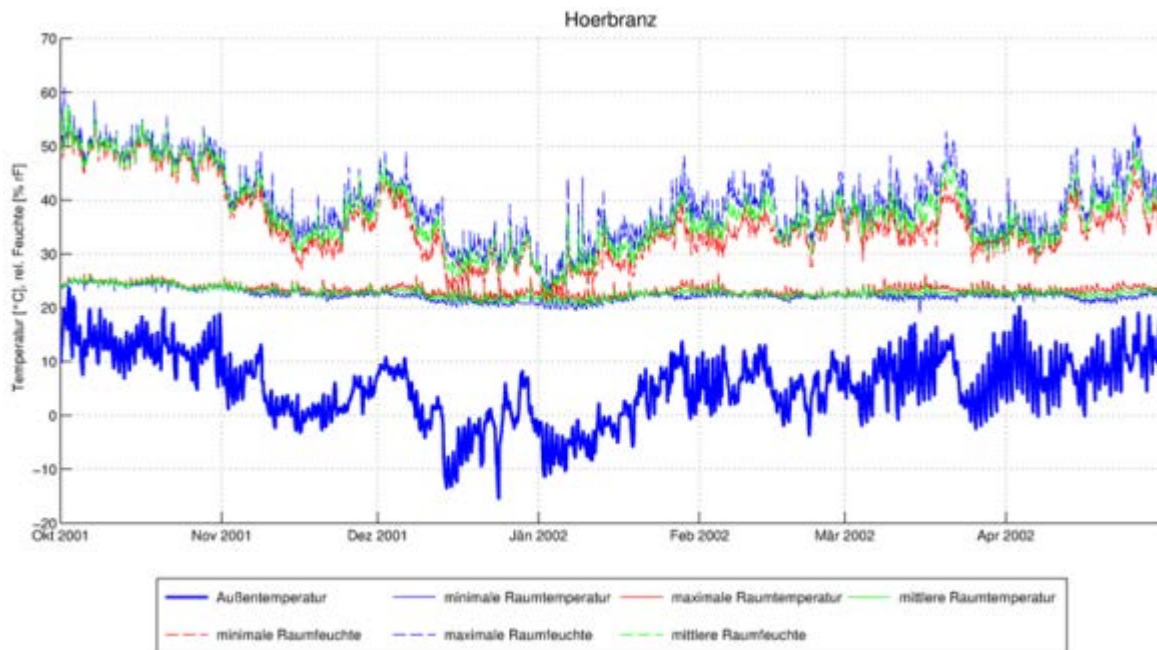
Abbildung 79: Hörbranz, Heizperiode (1. Oktober – 30. April) Stundenmittelwerte
