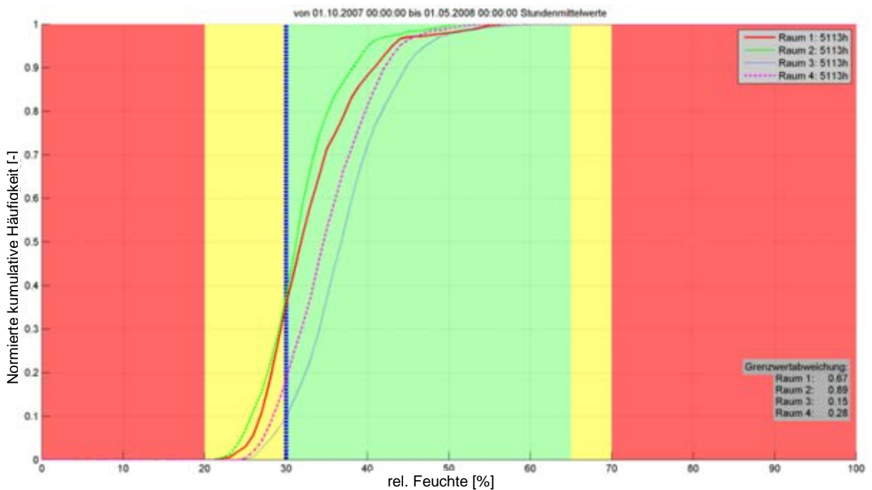
Abbildung 99: Mühlgweg, Heizperiode (1. Oktober – 30. April), Werte rechts oben stellen die Gesamtstundenzahl der gemessenen Werte für jeden Raum dar, Zielwertabweichung stellt die Summe der Unterschreitung der Grenze von 30 %-rF dar
