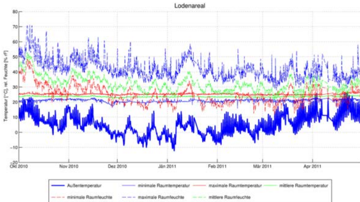
Abbildung 100: Lodenareal, Heizperiode (1. Oktober – 30. April) Stundenmittelwerte
