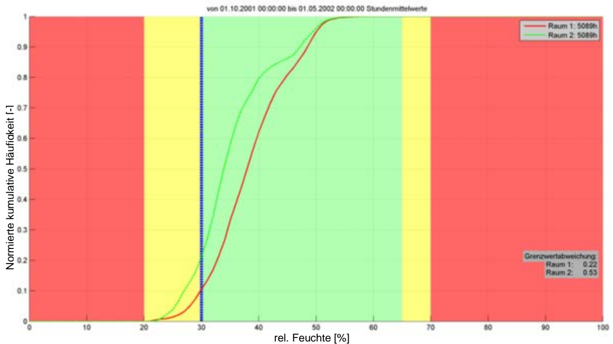
Abbildung 84: Hörbranz, Heizperiode (1. Oktober – 30. April), Werte rechts oben stellen die Gesamtstundenzahl der gemessenen Werte für jeden Raum dar, Zielwertabweichung stellt die Summe der Unterschreitung der Grenze von 30 %-rF dar
