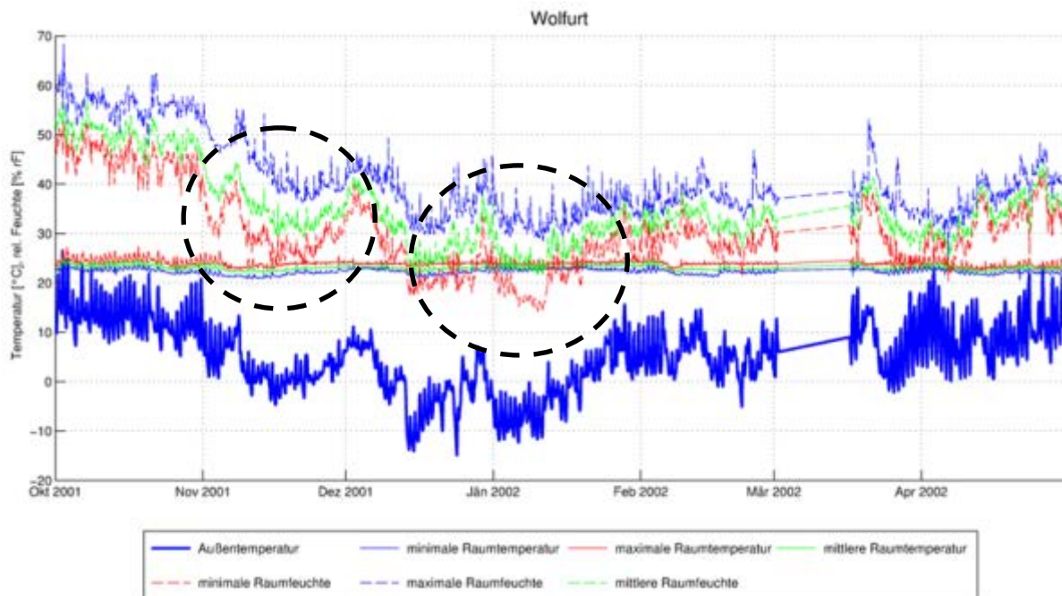
Abbildung 85: Wolfurt, Heizperiode (1. Oktober – 30. April) Stundenmittelwerte
