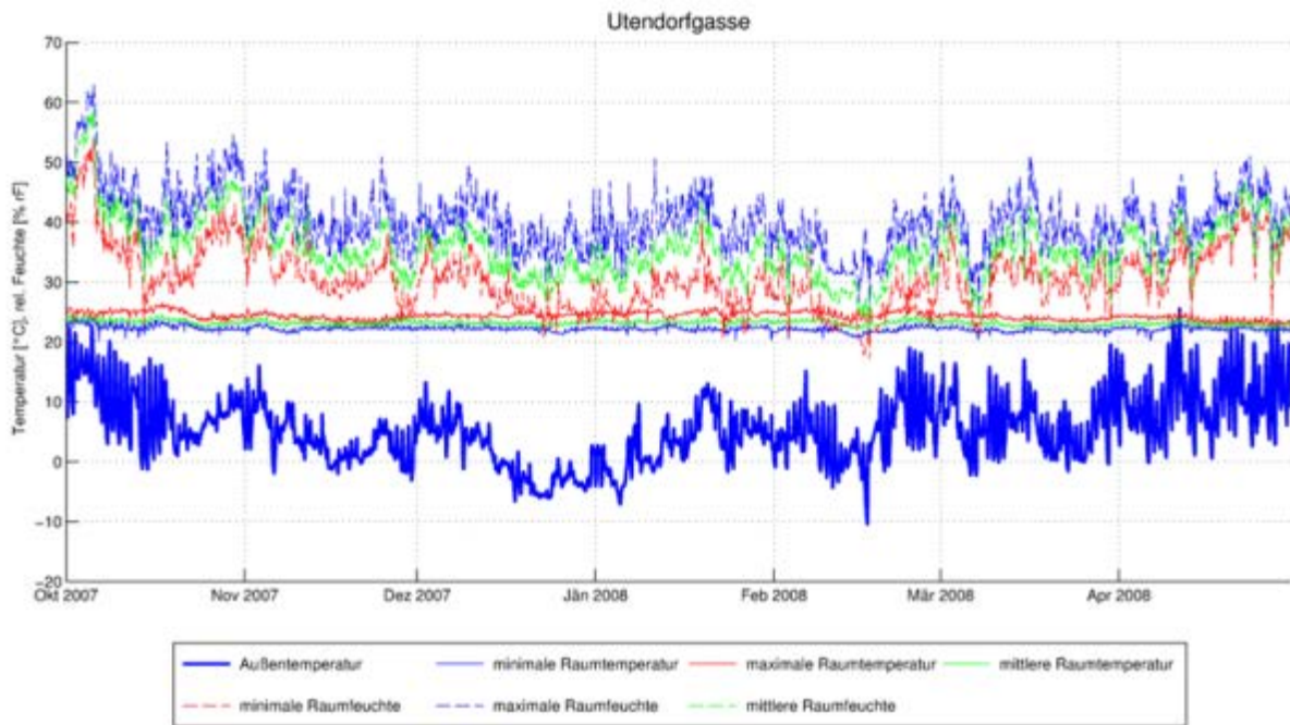
Abbildung 73: Utendorfasse, Heizperiode (1. Oktober – 30. April) Stundenmittelwerte
