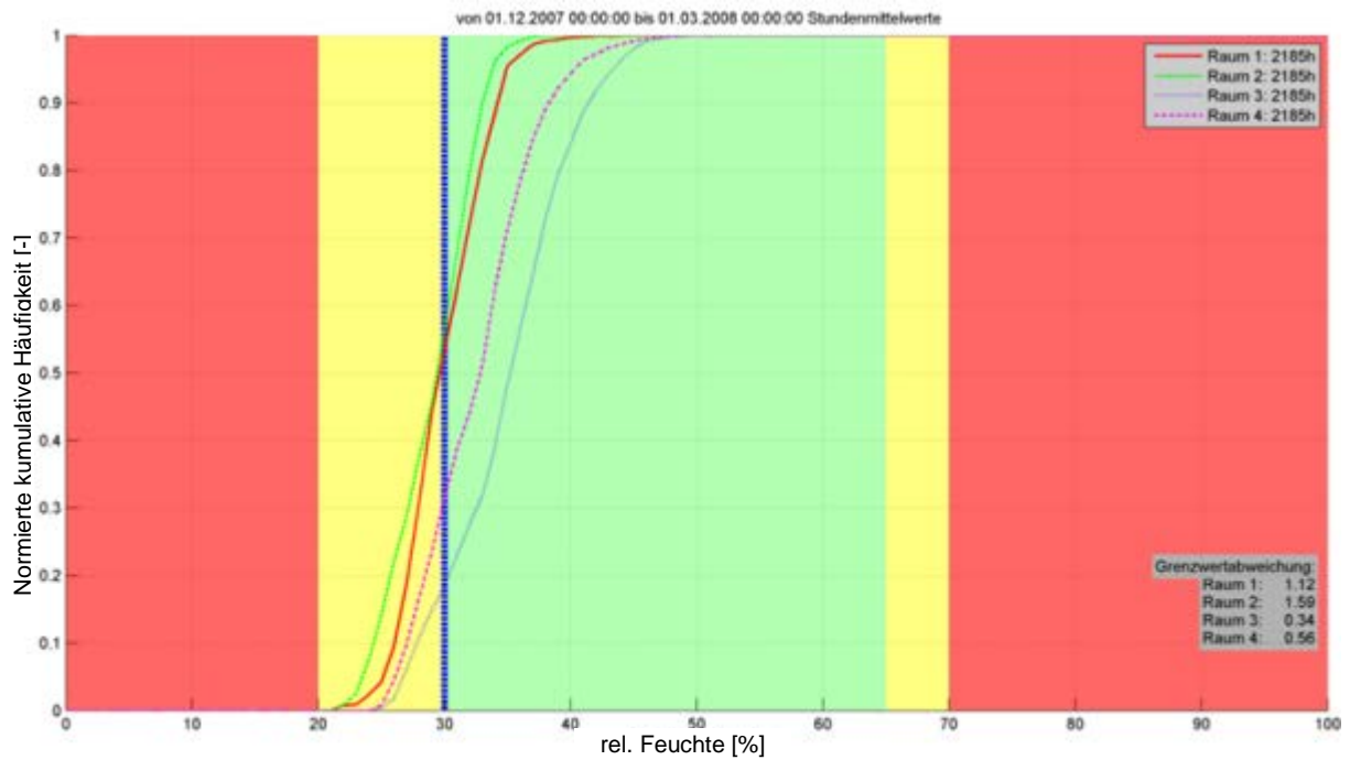
Abbildung 98: Mühlgweg, Kernwinter (1. Dezember – 28. Februar), Werte rechts oben stellen die Gesamtstundenzahl der gemessenen Werte für jeden Raum dar, Zielwertabweichung stellt die Summe der Unterschreitung der Grenze von 30 %-rF dar
